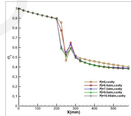
(d) Total pressure recovery
