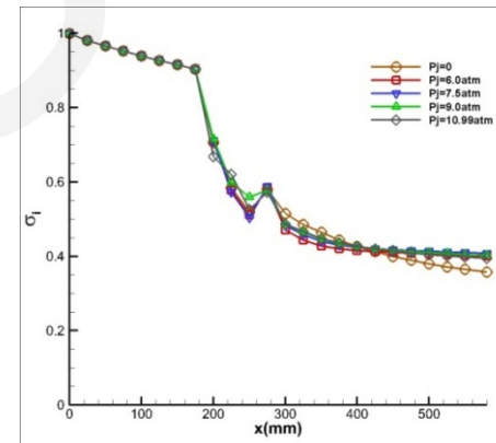
(d) Total pressure recovery
