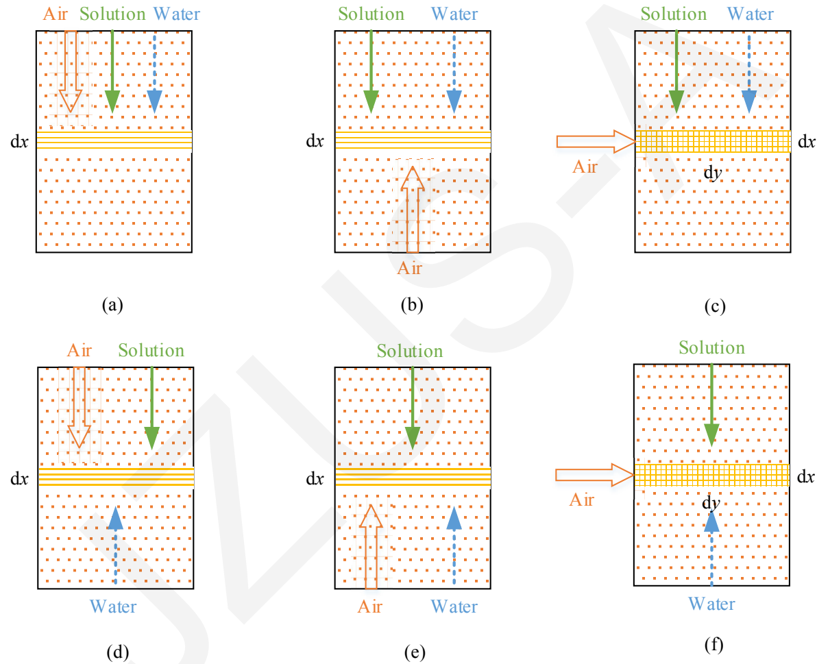
Fig. 1 Physical models of internally-cooled dehumidifiers (a) Pa.- I ; (b) Co.- I ; (c) Cr.- I ; (d) Pa.- II ; (e) Co.- II ; (f) Cr.- II
