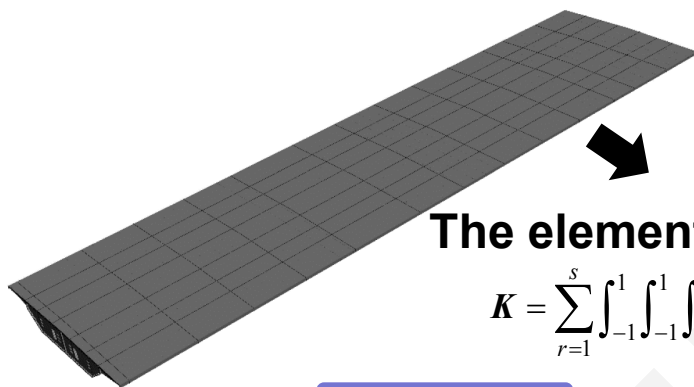
A-FEM model
