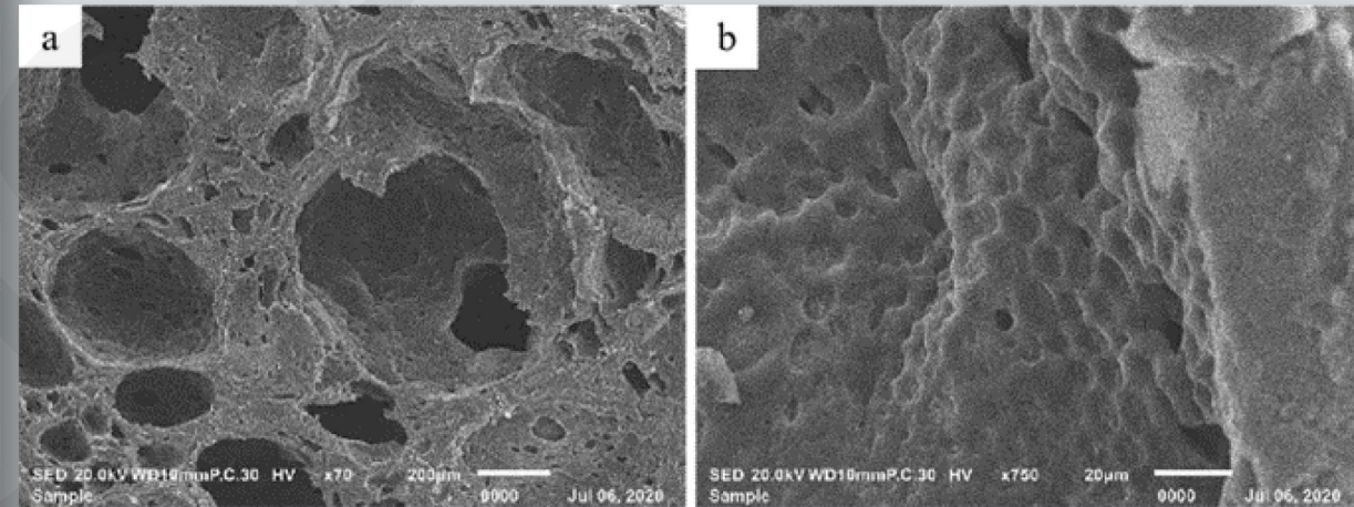
Fig. 3 SEM Images of SiO 2 @IBR
